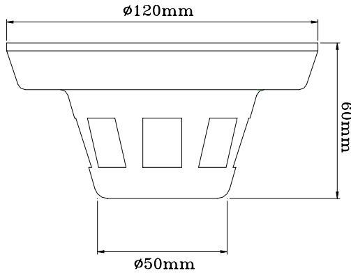
Yandan Görünüş
